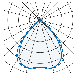
90° optic
