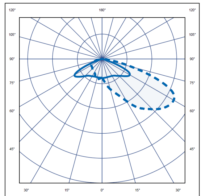
L8 Optic
