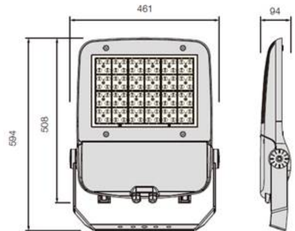
L8 Optic
