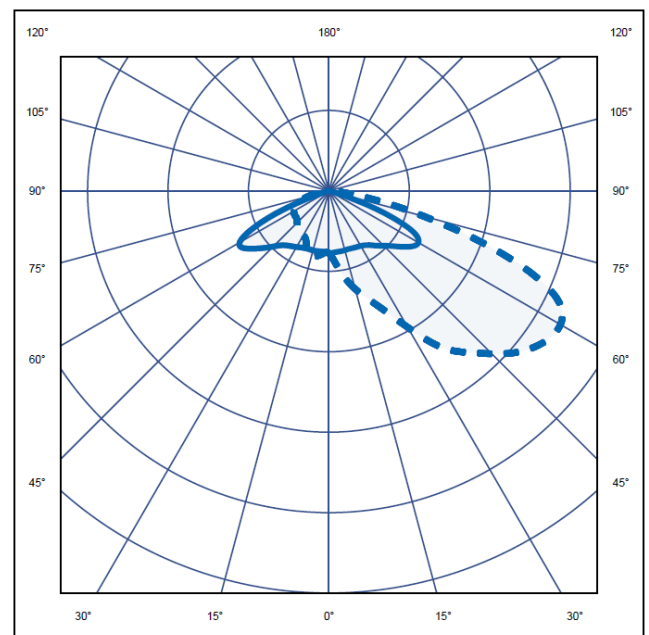
L8 Optic
