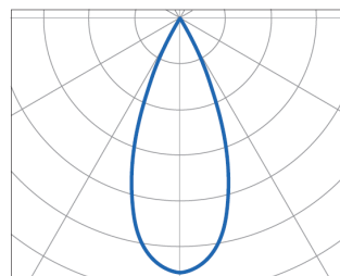
50° reflector
