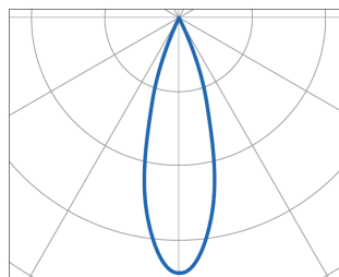
25° reflector
