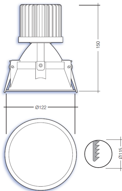
50° reflector
